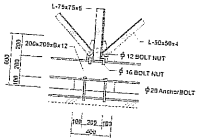
A 기초상세도 SCALE: NONE
