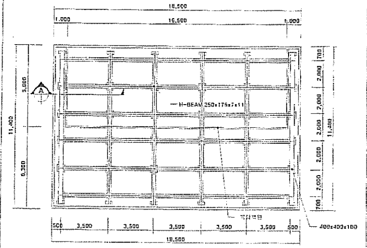
강철 옥상바닥 하부구조도 SCALE 1/300
