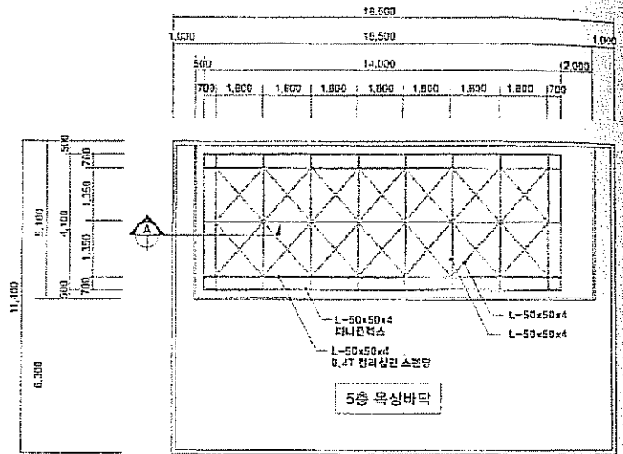
평면도 SCALE: 1/50
