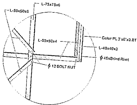
B 부분상세도 SCALE: NONE
